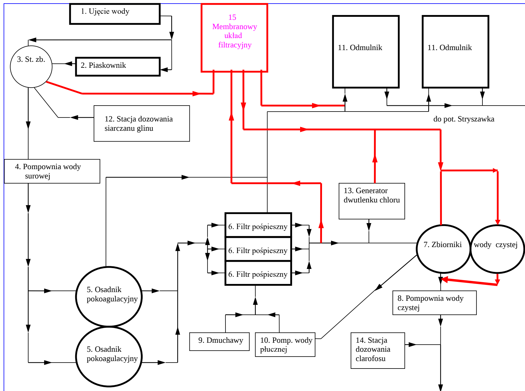
Schemat technologiczny Stacji Uzdatniania Wody
